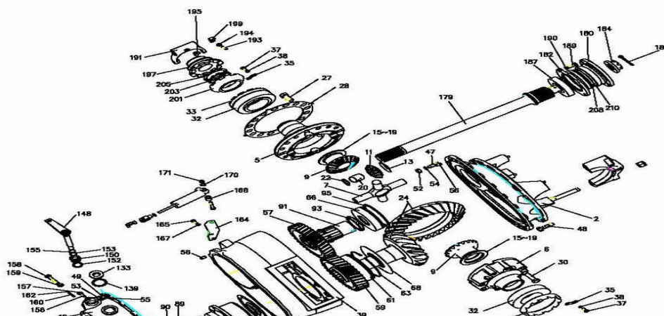
中桥驱动装置
