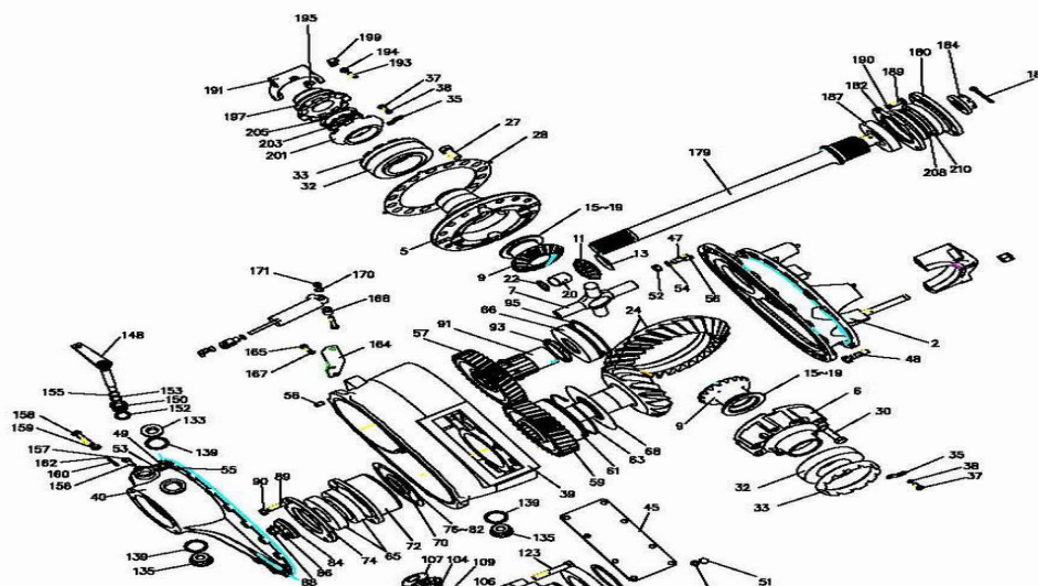
中桥驱动装置
