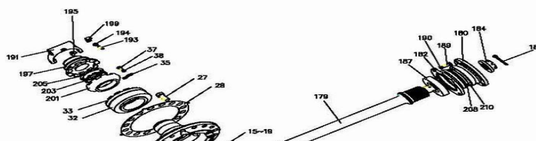
中桥驱动装置
