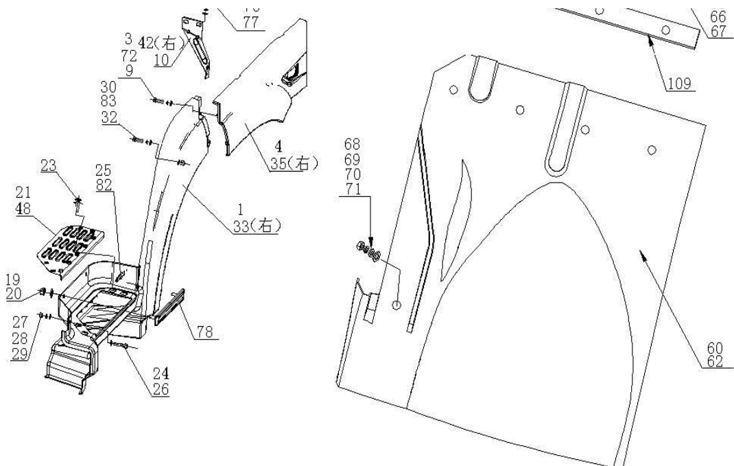
1. 34 中长驾驶室新造型翼子板/Fender
