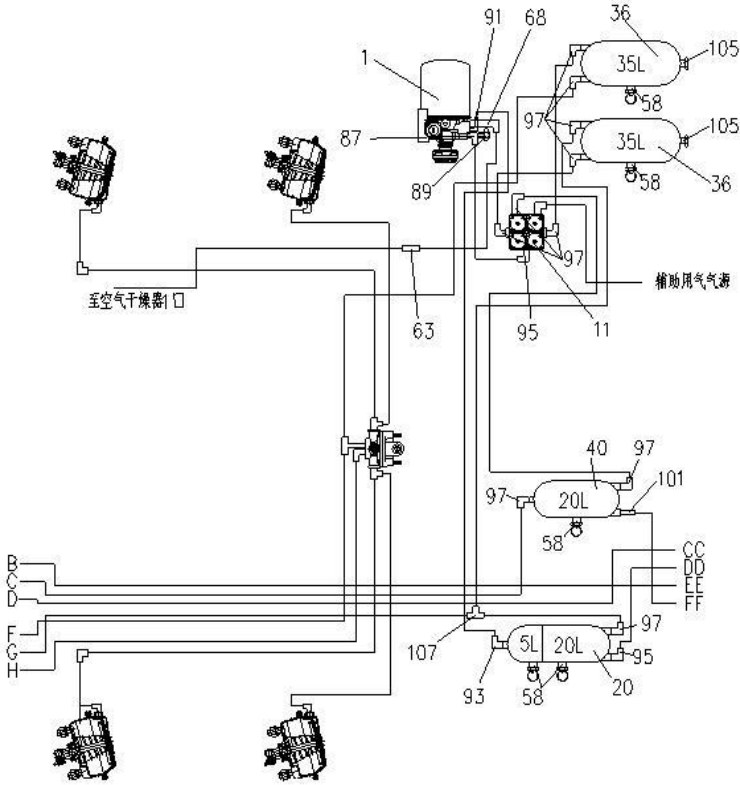
8.18 HW8X4底盘制动装置/Chassis Brake Device
