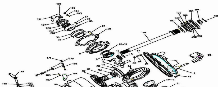
中桥驱动装置
